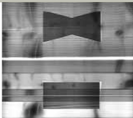
Röntgenaufnahme (Draufsicht/Seitenansicht) eines Dübelbalkens mit Hartholzdübel
